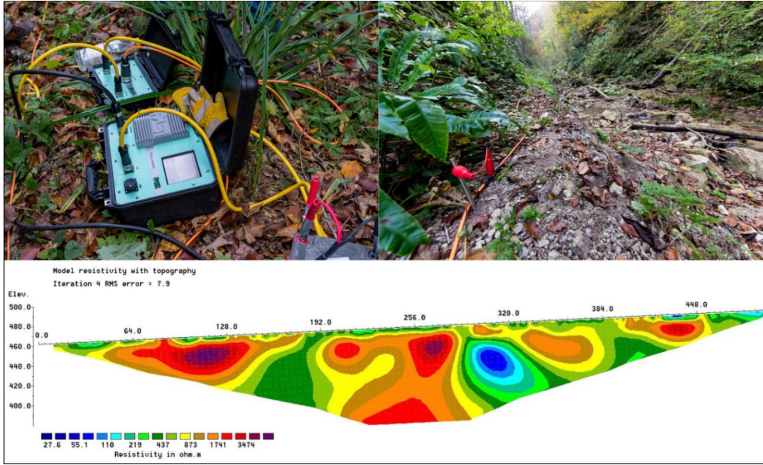
Izgled postavljene opreme na terenu (gore) i interpretirani rezultati istraživanja (dolje)
